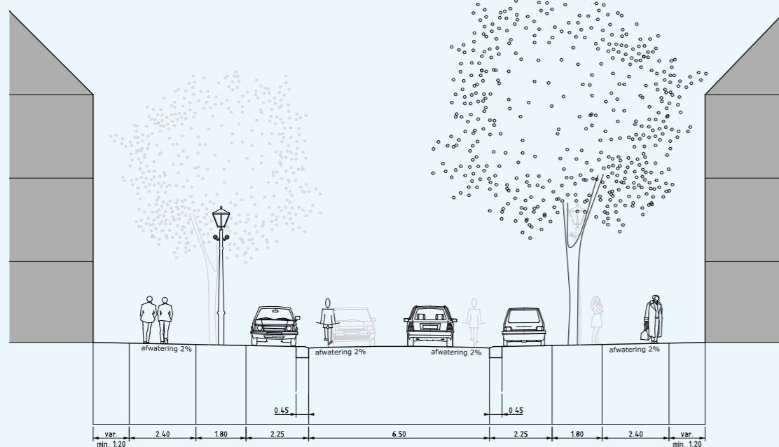
Frederik Hendriklaan - dwarsprofiel
