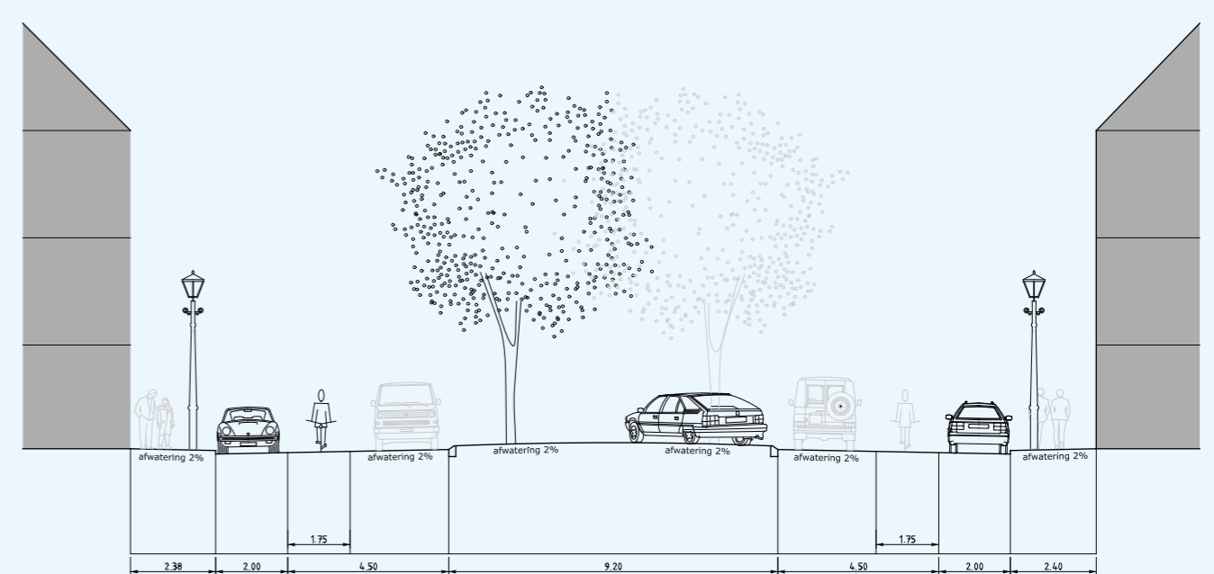
Willem de Zwijgerlaan - dwarsprofiel
